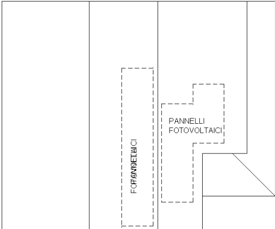
PIANO COPERTURA 4
